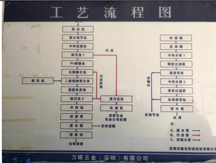
防治污染设施工艺流程图
